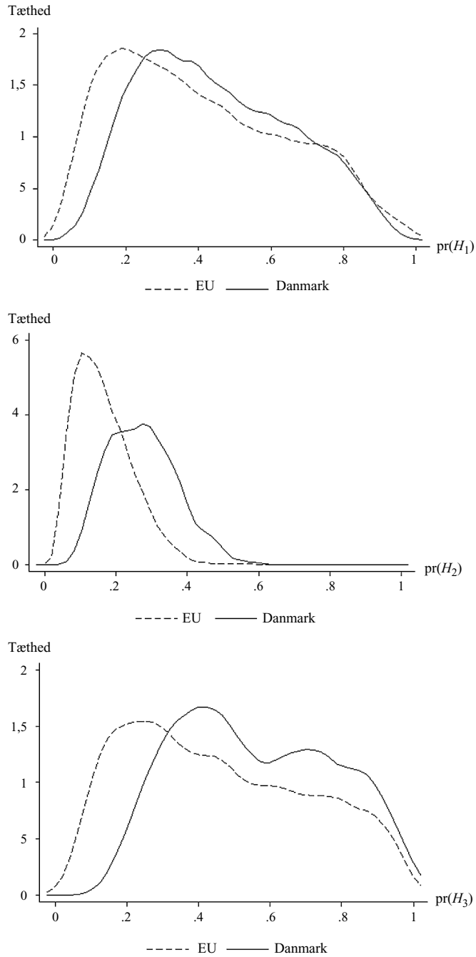
Figur 6.1. Kernel tætheder for predikerede sandsynligheder.
